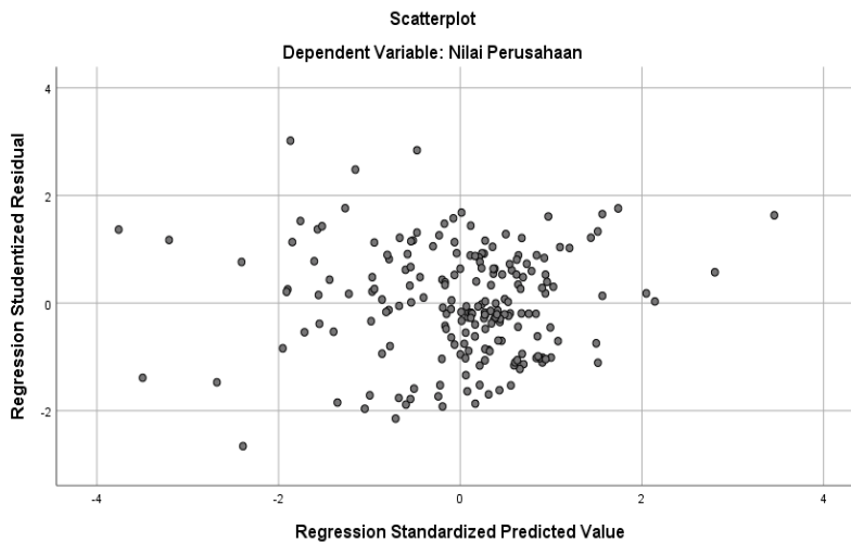
Gambar 1 Uji Heterokedastisitas
