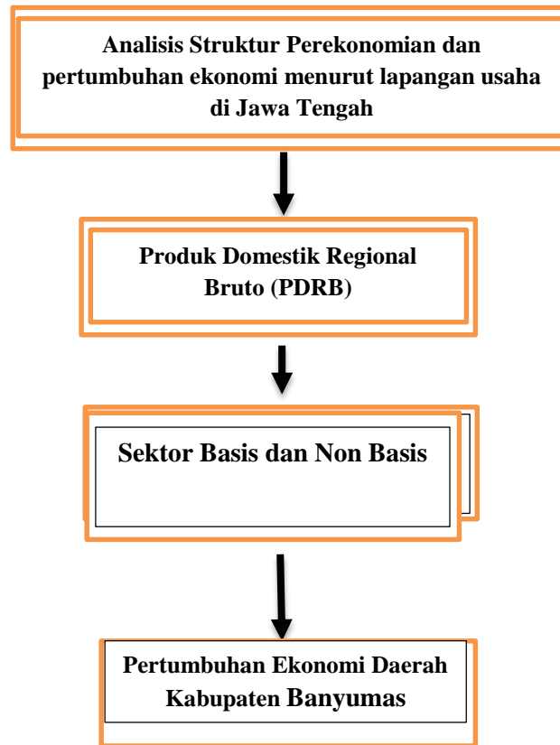
Gambar 1. Kerangka Penelitian
