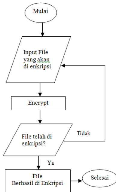
Gambar 1. Proses Enkripsi
