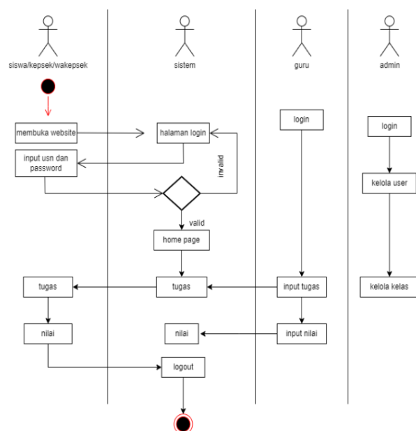
Gambar 5. Flow Map Sistem diusulkan
